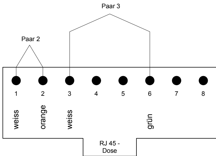
linke Buchse Ethernet
