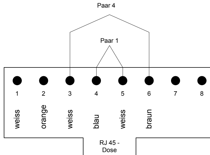
rechte Buchse Telefon
